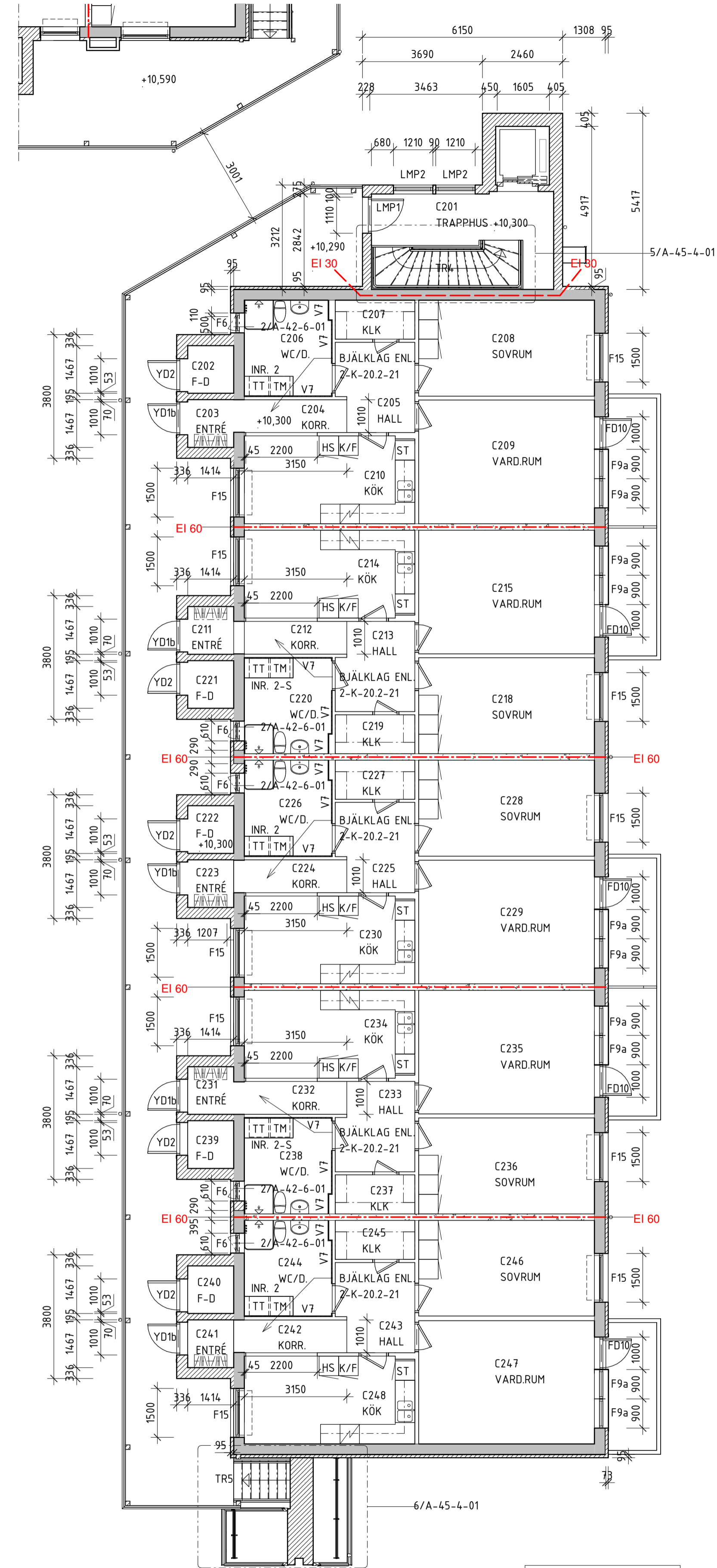
HUS C PLAN 1TR 1 : 100
